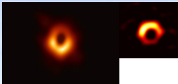
Vlevo na obrázku je numerická simulace, a nalevo se nachází fotografie černé díry.
